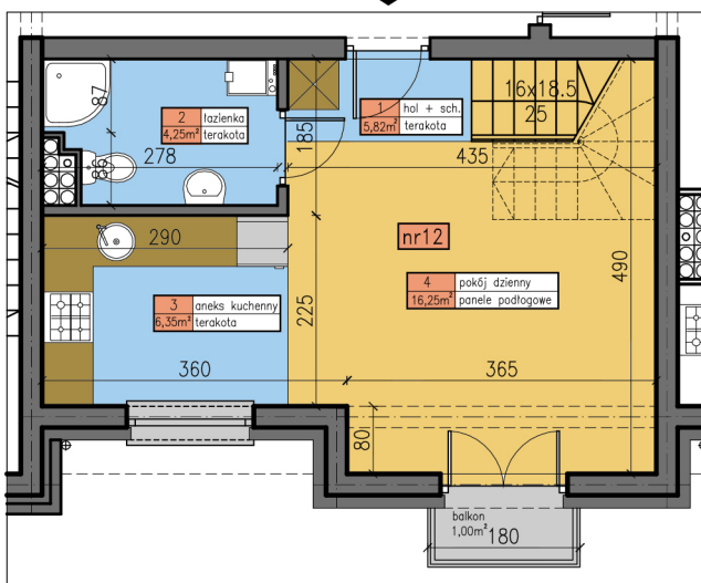
KONDYGNACJA 3
