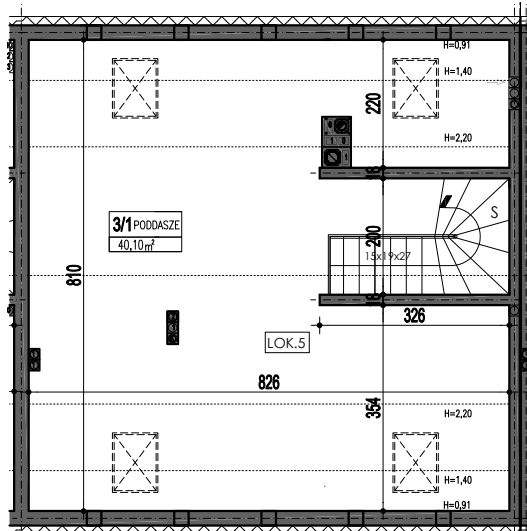
RZUT PODDASZA
