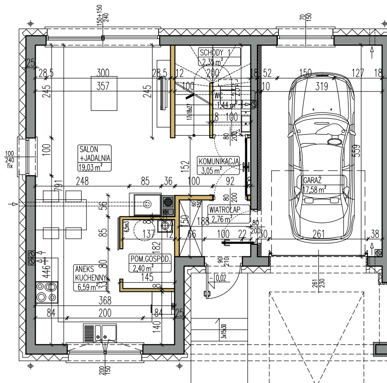
RZUT PARTERU
