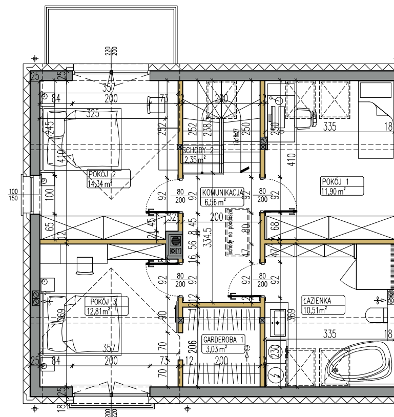
RZUT PODDASZA
