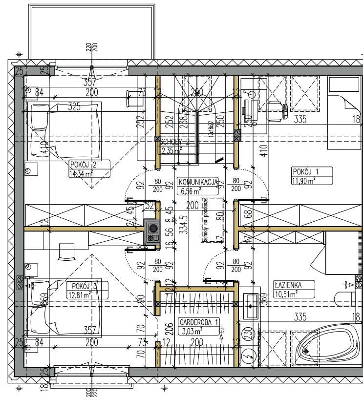
RZUT PODDASZA
