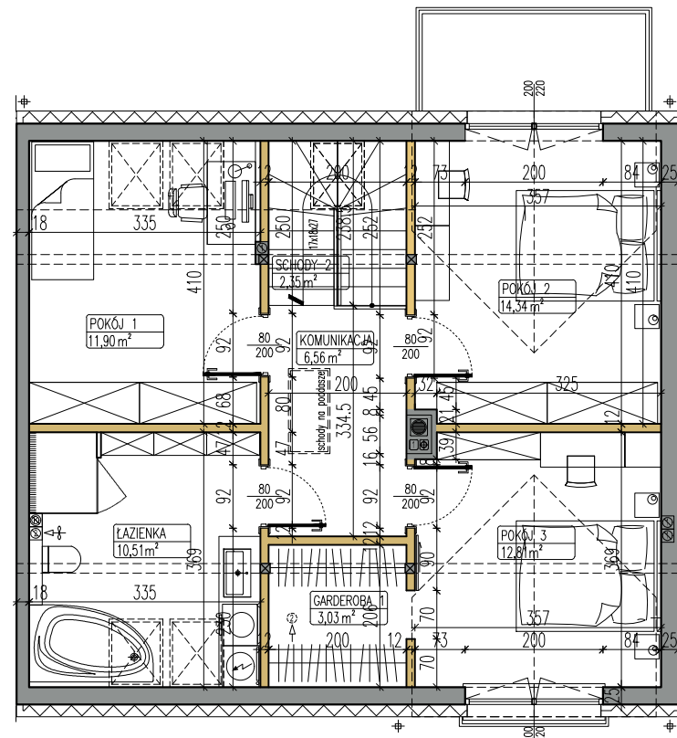
RZUT PODDASZA
