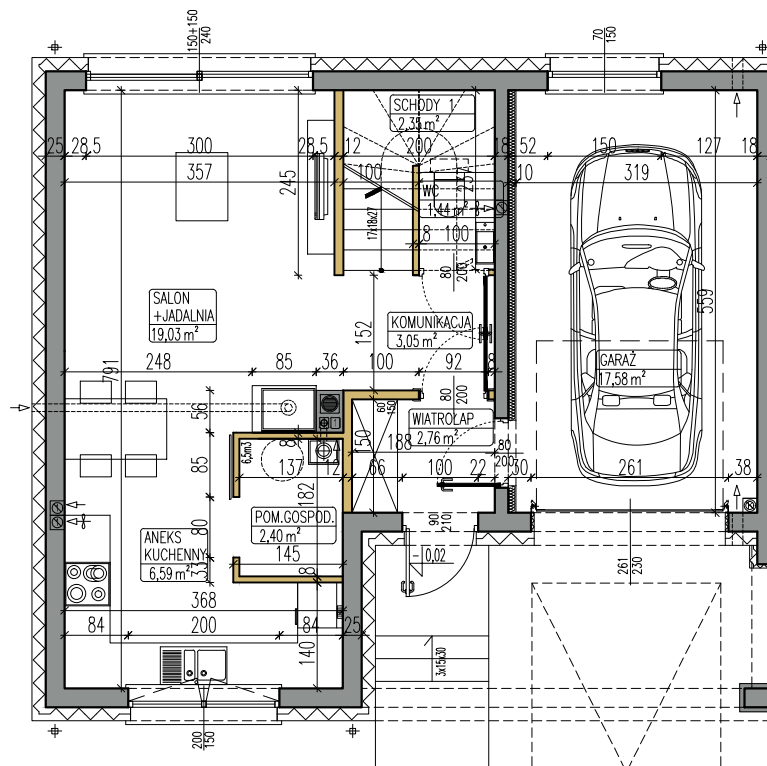
RZUT PARTERU
