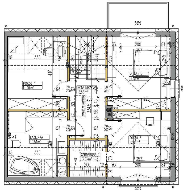
RZUT PODDASZA
