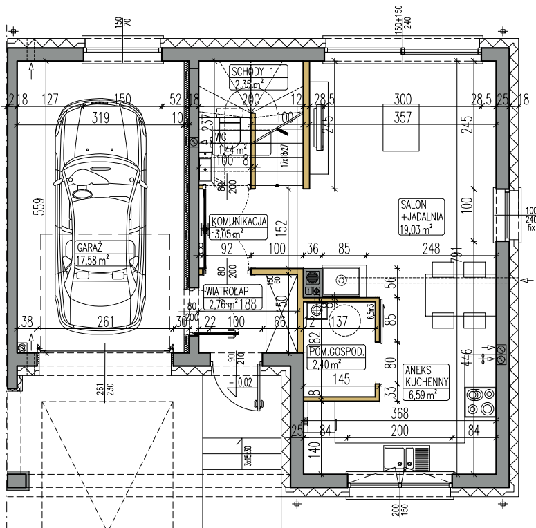
RZUT PARTERU
